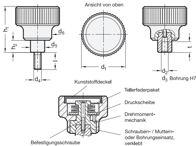
GN 3663-mit Gewindebolzen
